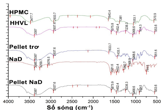
Hình 4. Phổ hồng ngoại của NaD, HPMC, hỗn hợp vật lý (HHVL), pellet trống và pellet NaD
